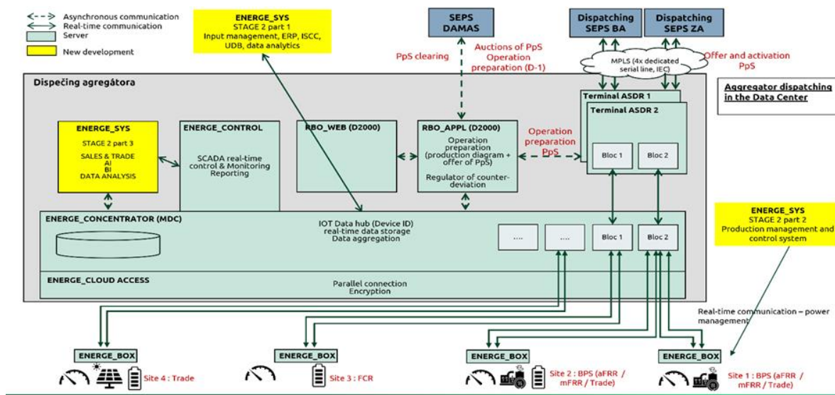
Obrázok 3: Konceptuálne technické riešenie a komunikačná infraštruktúra
